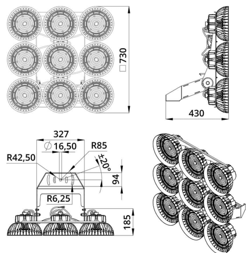
Габаритный чертёж
