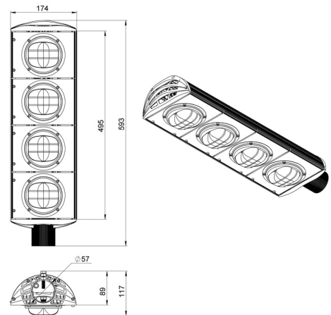
Габаритный чертёж
