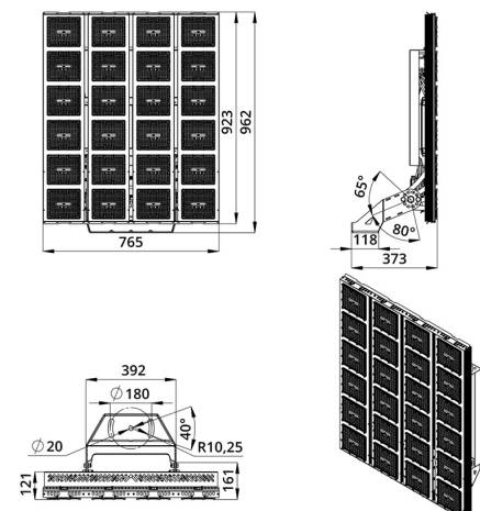
Габаритный чертеж
